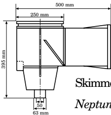
Neptun ABS múanyag és rozsdamentes acél fölözőedény
