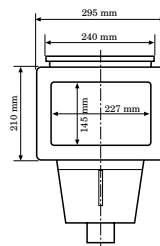
Skimmer Neptun DLHY
