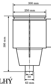
Neptun Lang fölözőedény
