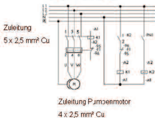
Schaltplan Pumpe dreiphasig
