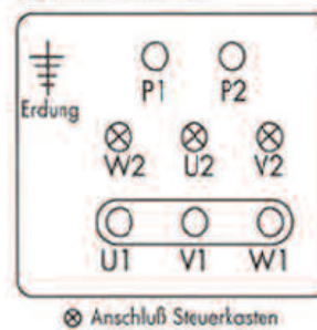
Pumpenschaltkasten 400 V
