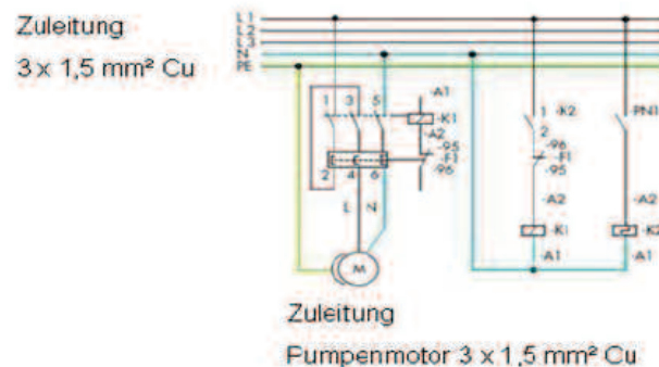
Schaltplan Pumpe 2 kW / 230 V / 9,8 A
